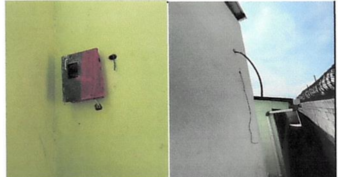
Foto 4: reparación de cableado electrico y sustitución de conductos, cambio de caja para flipones para la cometida electrica.
